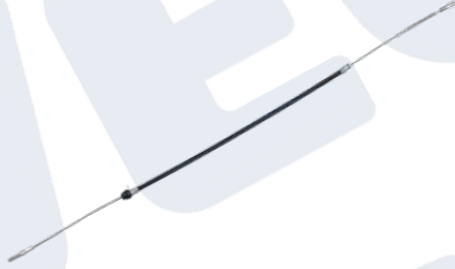
EL FREN HALATI ARKA SAĞ SOL ORJİNAL NO : 28150 MODEL : M 23 UZUNLUK : 1.170 MM.
