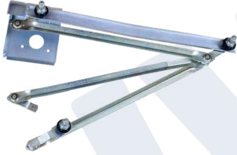
SİLECEK MEKANİZMASI KOMPLE ORJİNAL NO : 8392 MODEL : 65 85
