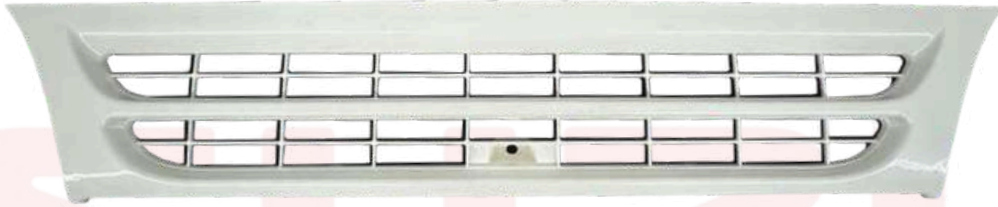
ÖN PANJUR (DÜBELLİ) ORJİNAL NO : 8970789532 MODEL : NPR 66
